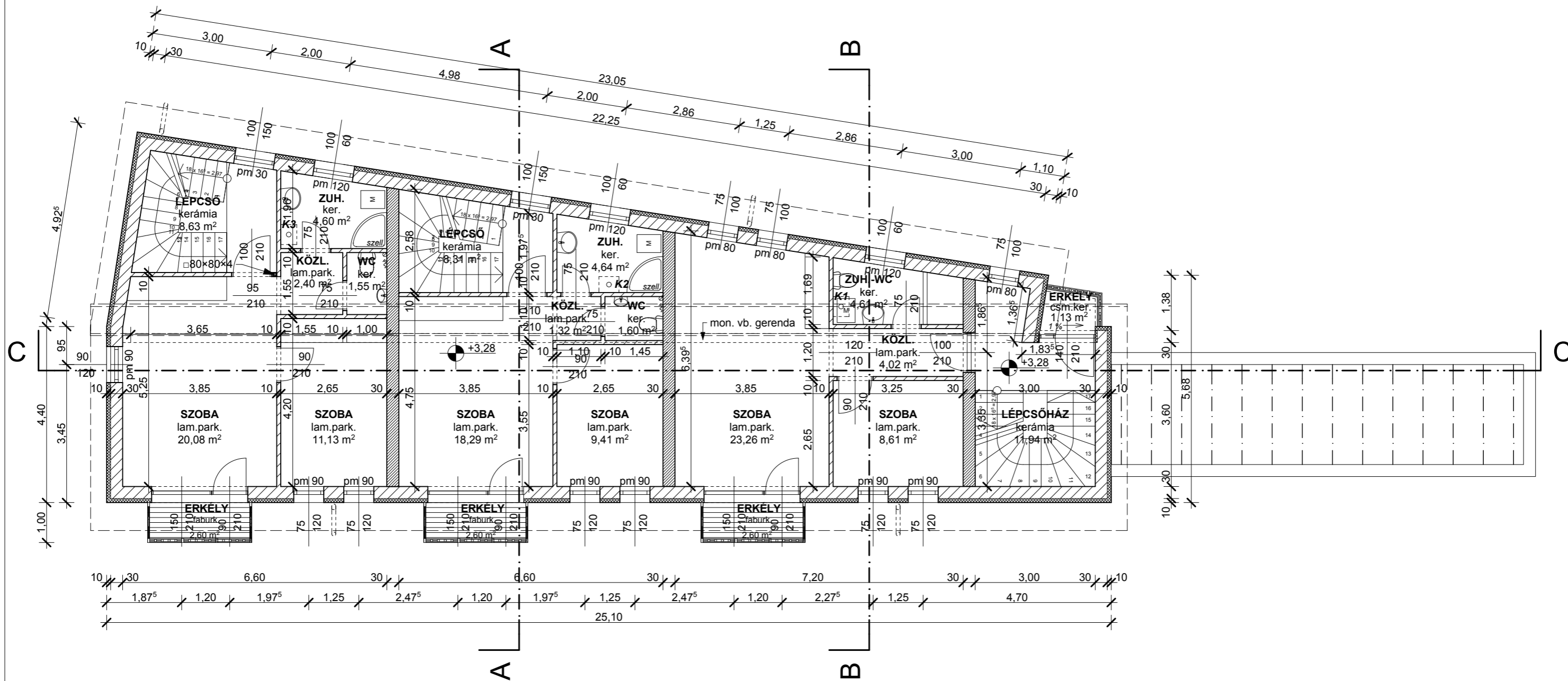
EMELETI ALAPRAJZ M 1:100
